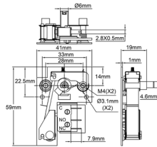
Ohne Verbindungsblock
